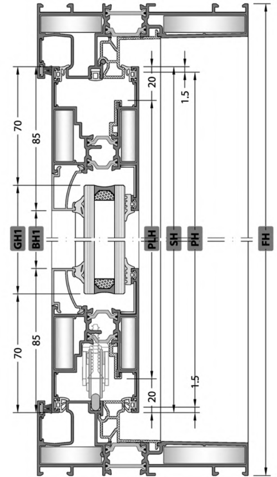
A-A SECTION / A-A KESİTİ
