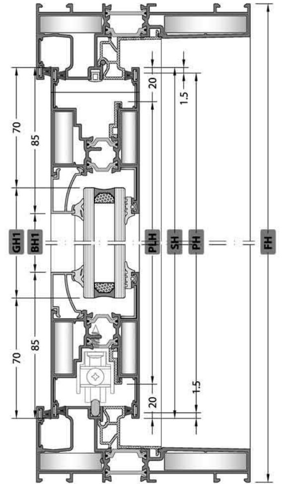
A-A SECTION / A-A KESİTİ
