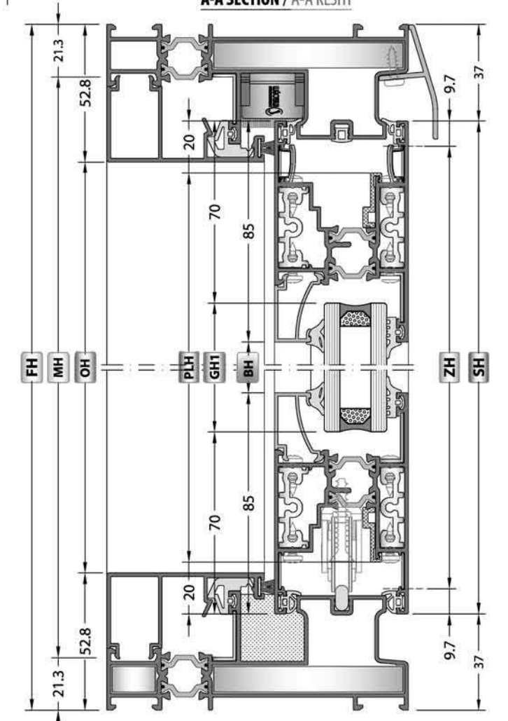
B-B SECTION / B-B KESİTİ
