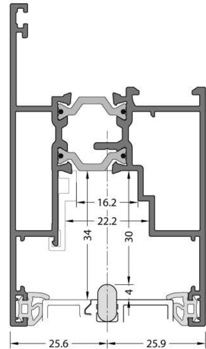
Univesal Lift & Slide Accesories Groove Universal Kaldır-Sür Aksesuar Kanalı
