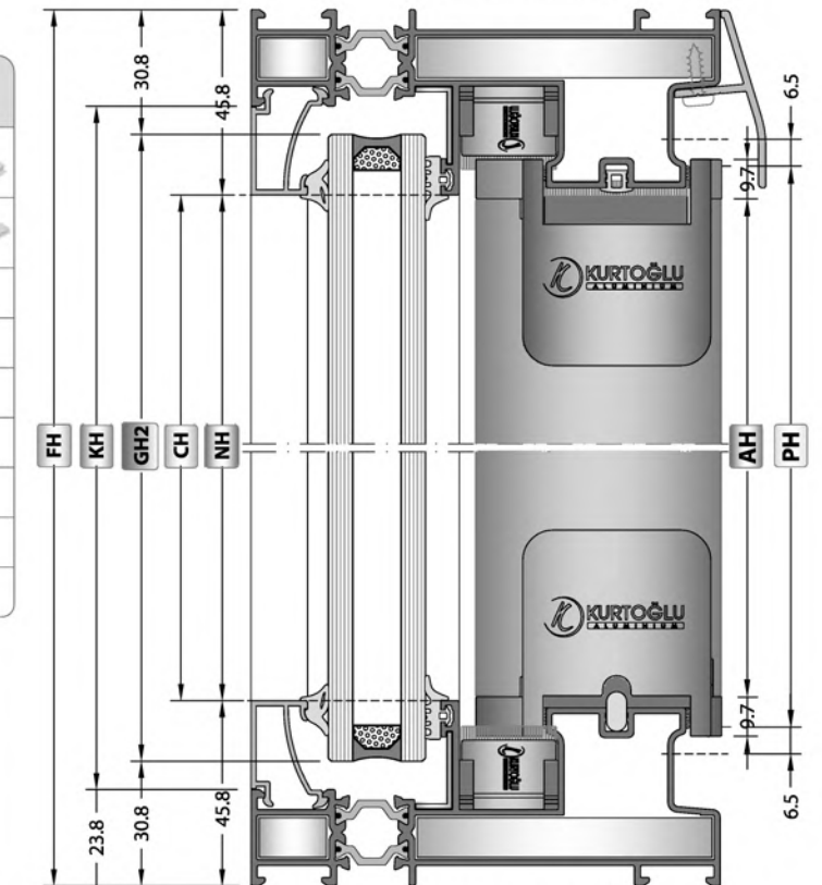
A-A SECTION / A-A KESİTİ
