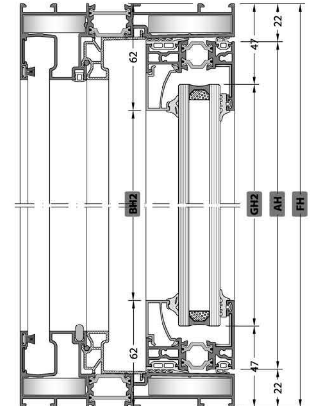
B-B SECTION / B-B KESİTİ
