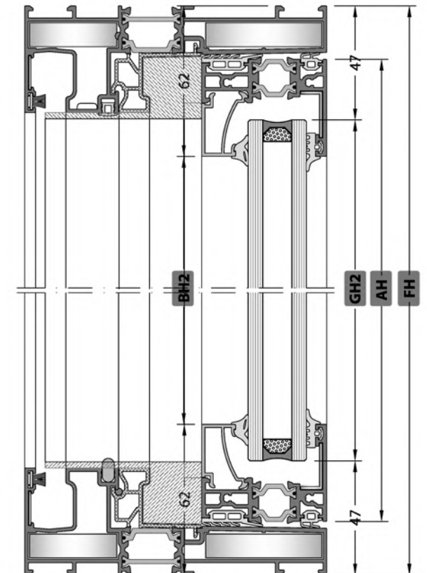
B-B SECTION / B-B KESİTİ
