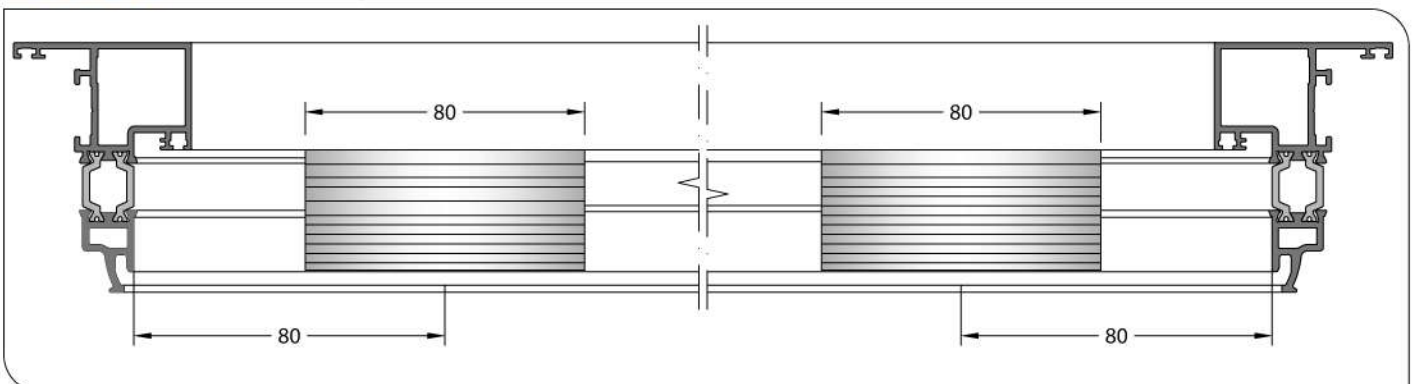
TOP VIEW / ÜST GÖRÜNÜŞ
