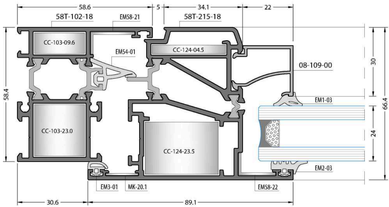
Exterior Window Sash Profile Details / Dışa Açılır Pencere Kanat Profil Detayları
