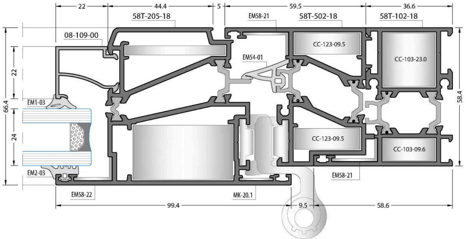
Inside Window and Outside Opening Door İçe Açılır Pencere ve Dışa Açılır Kapi
