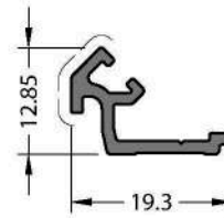
CODE / KOD 07-112-00 THEORETICAL WEIGHT kg/m TEORİK AĞIRLIK kg/m 0.148
