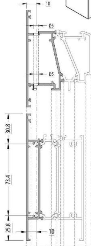
Screw Sizes / Vida Ölçüleri
