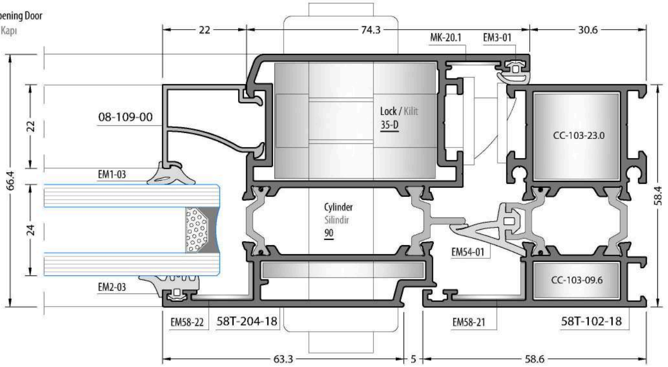
Inside Opening Door İçe Açılır Kapi
