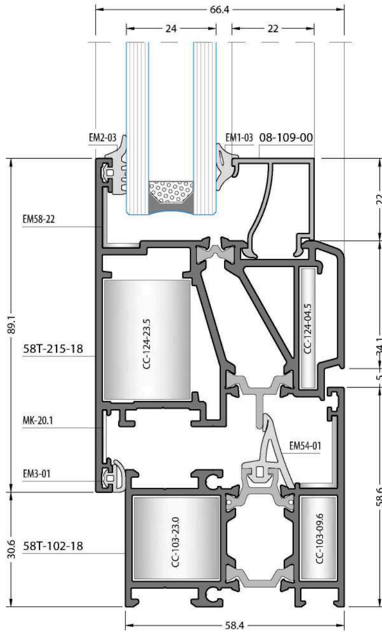
Exterior Window Sash Profile Details / Dışa Açılır Pencere Kanat Profil Detayları
