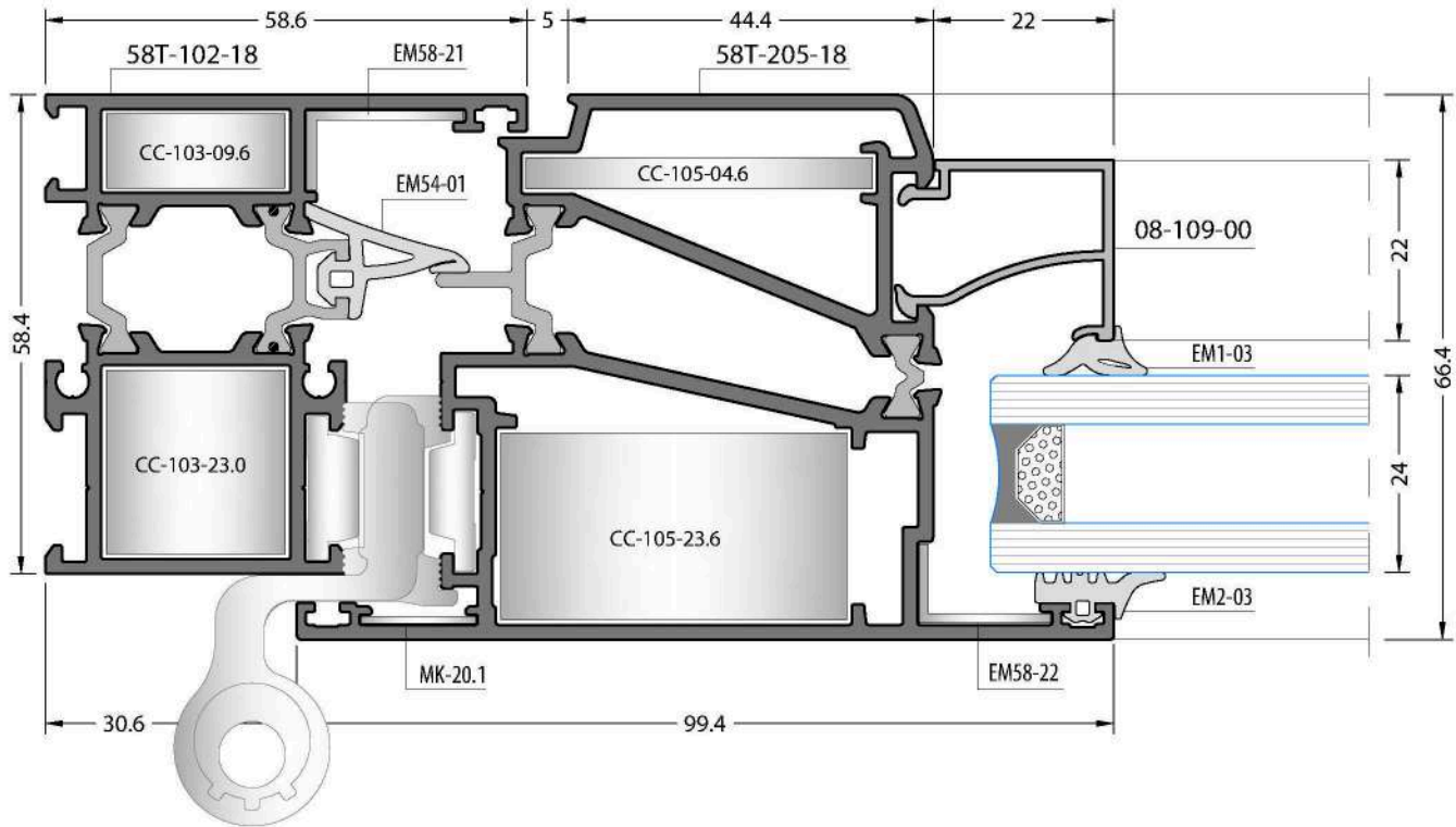
Outside Opening Door Dışa Açılır Kapi
