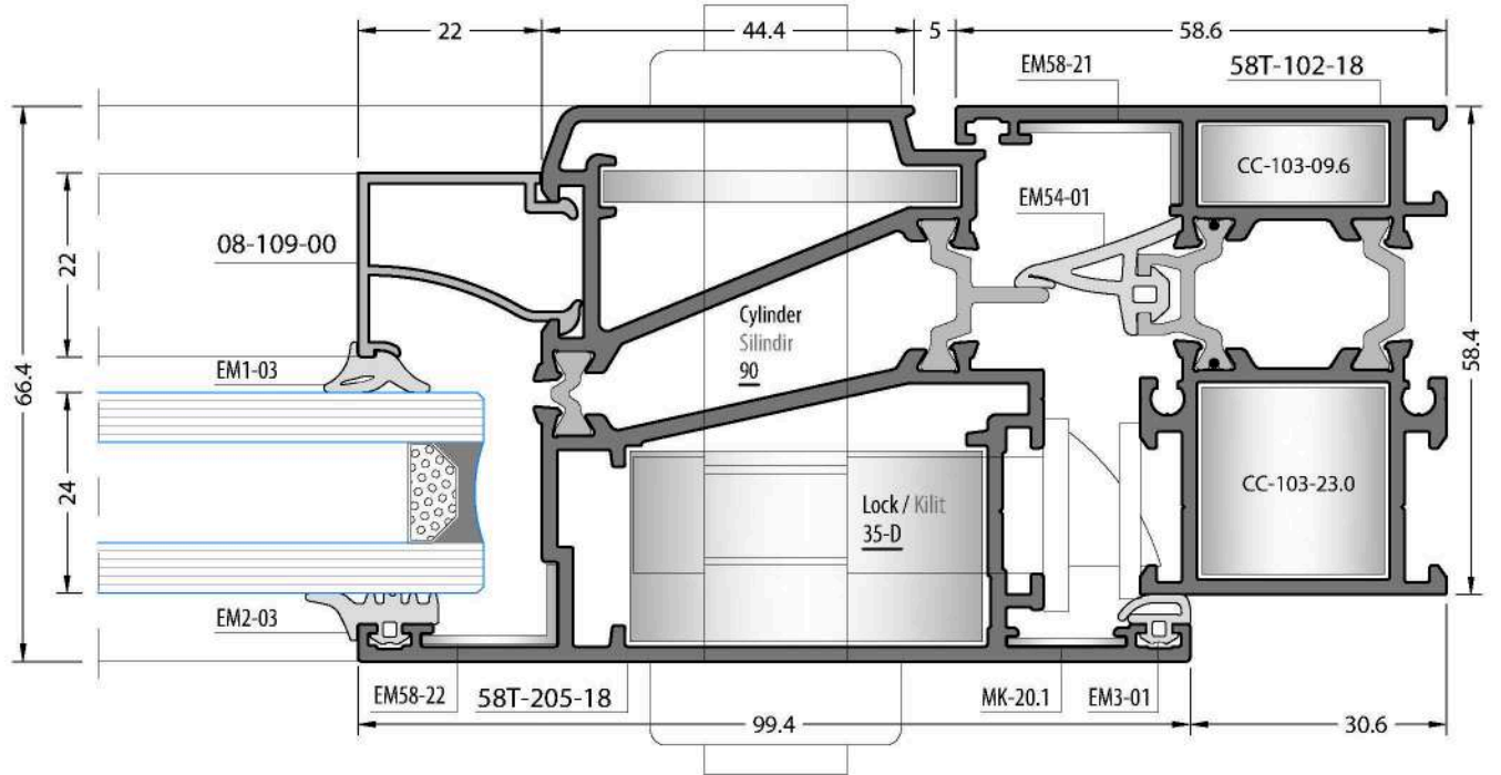
Outside Opening Door Dışa Açılır Kapi
