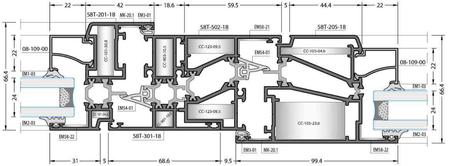
Inside Window and Outside Opening Door İçe Açılır Pencere ve Dışa Açılır Kapi
