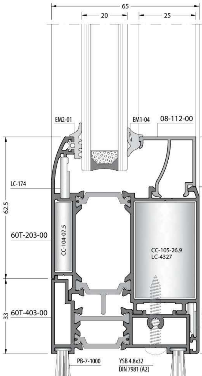
Inside Opening Door İçe Açılır Kapı
