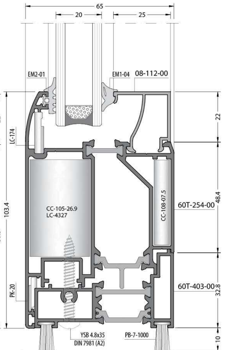
Outside Opening Door Dışa Açılır Kapı
