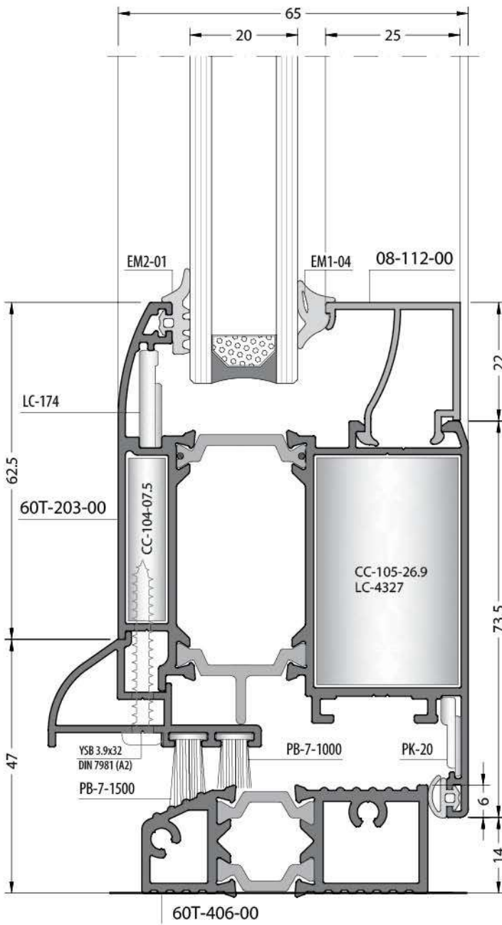
Inside Opening Door İçe Açılır Kapı
