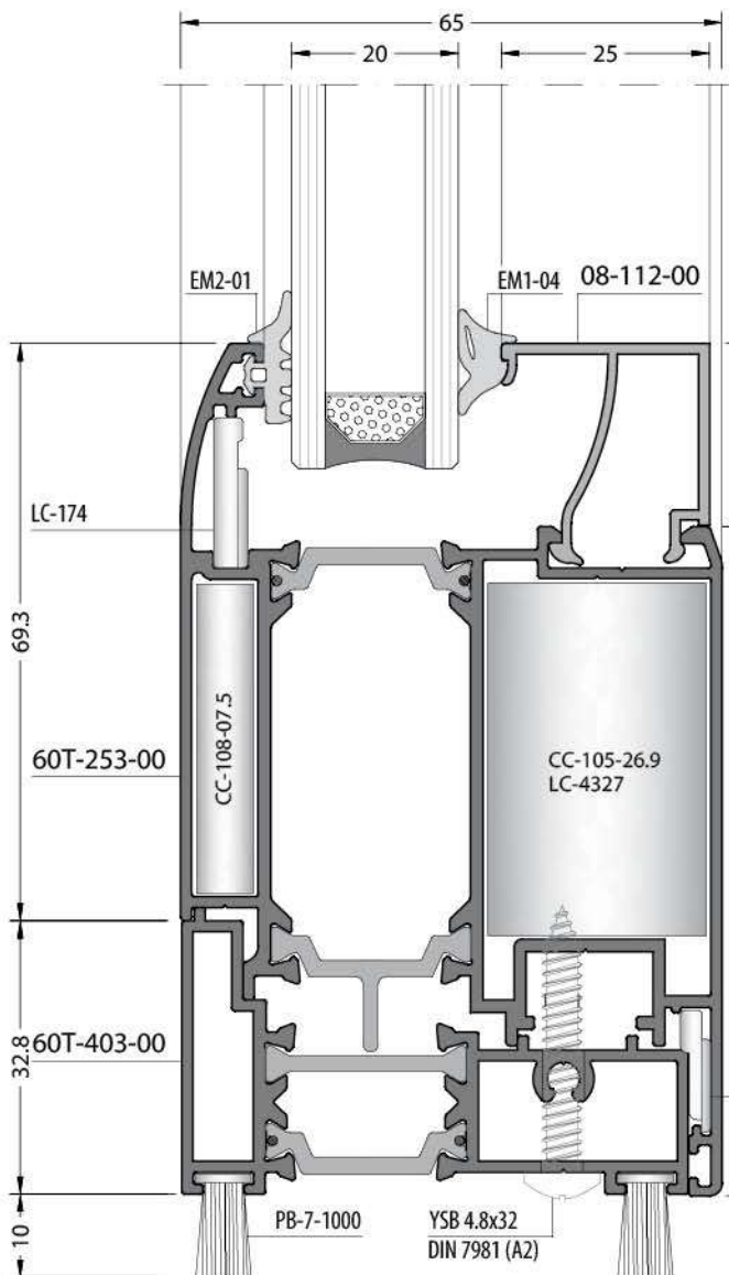
Inside Opening Door İçe Açılır Kapı
