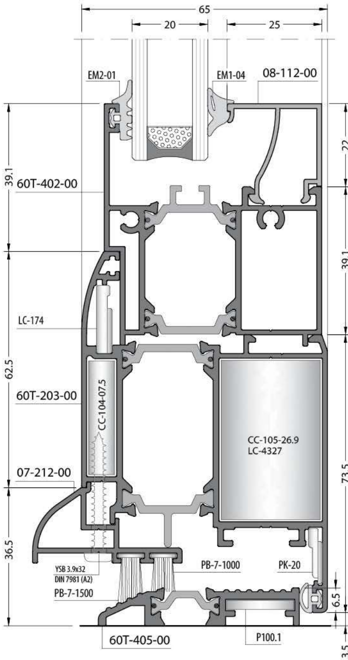
Inside Opening Door İçe Açılır Kapı
