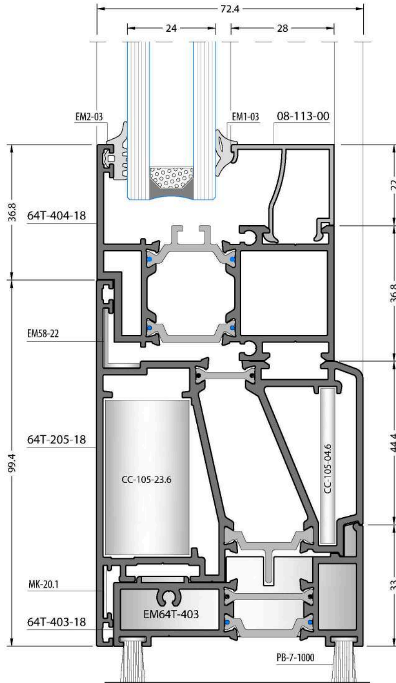
Outside Opening Door Dışa Açılır Kapi
