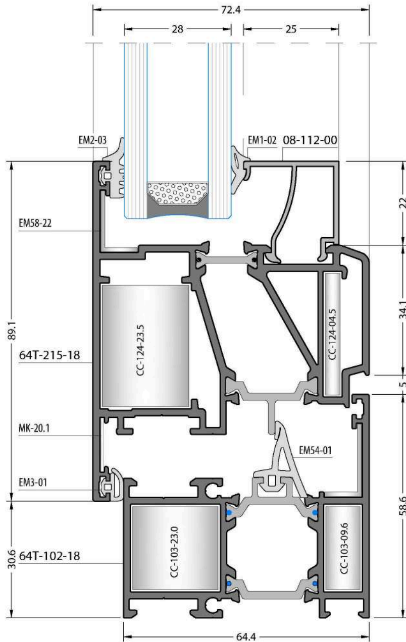
Exterior Window Sash Profile Details / Dışa Açılır Pencere Kanat Profil Detayları
