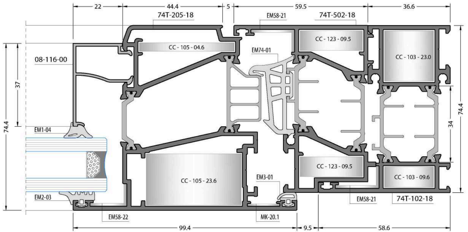
Outside Opening Door Dışa Açılır Kapı
