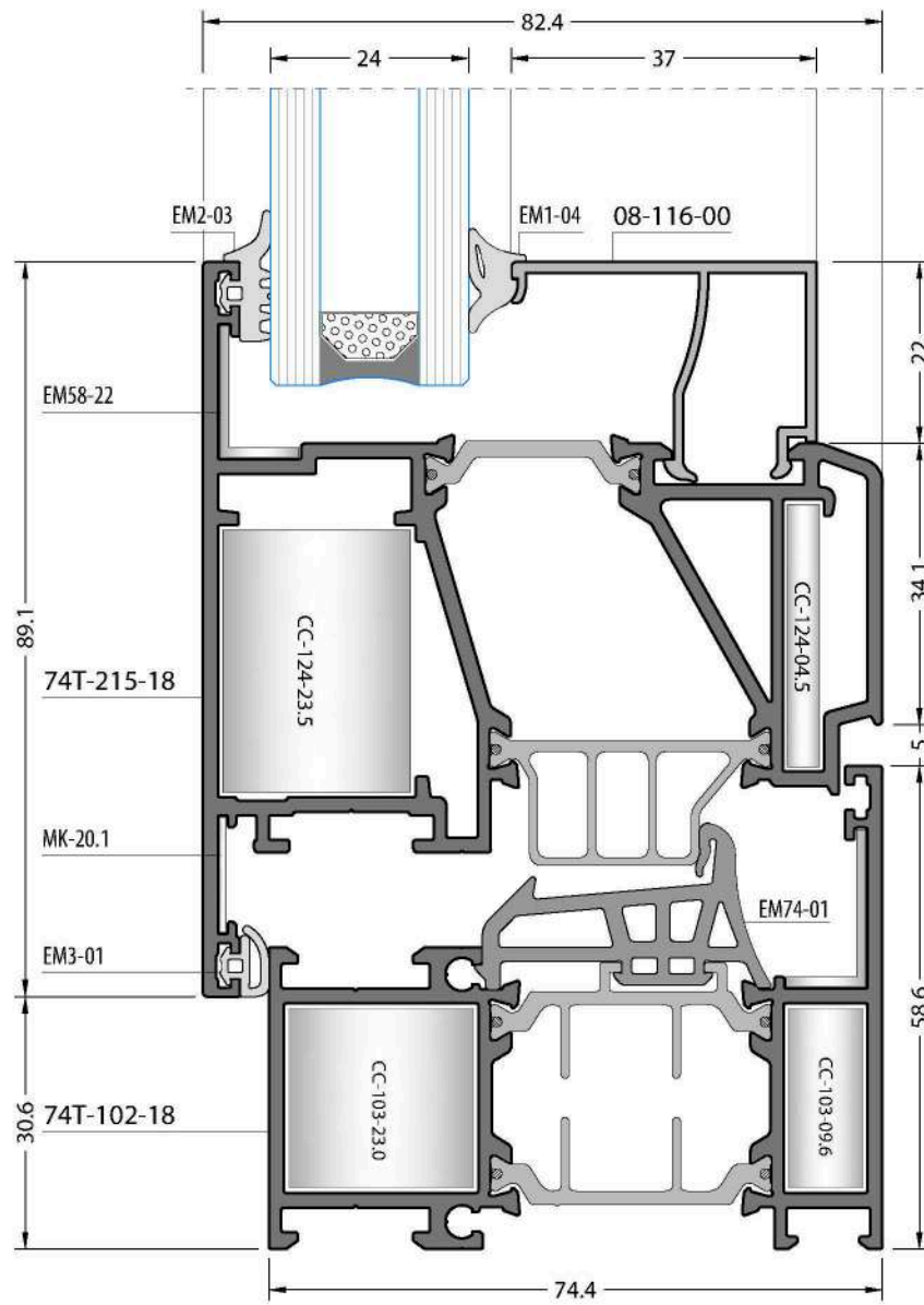
Exterior Window Sash Profile Details / Dışa Açılır Pencere Kanat Profil Detayları
